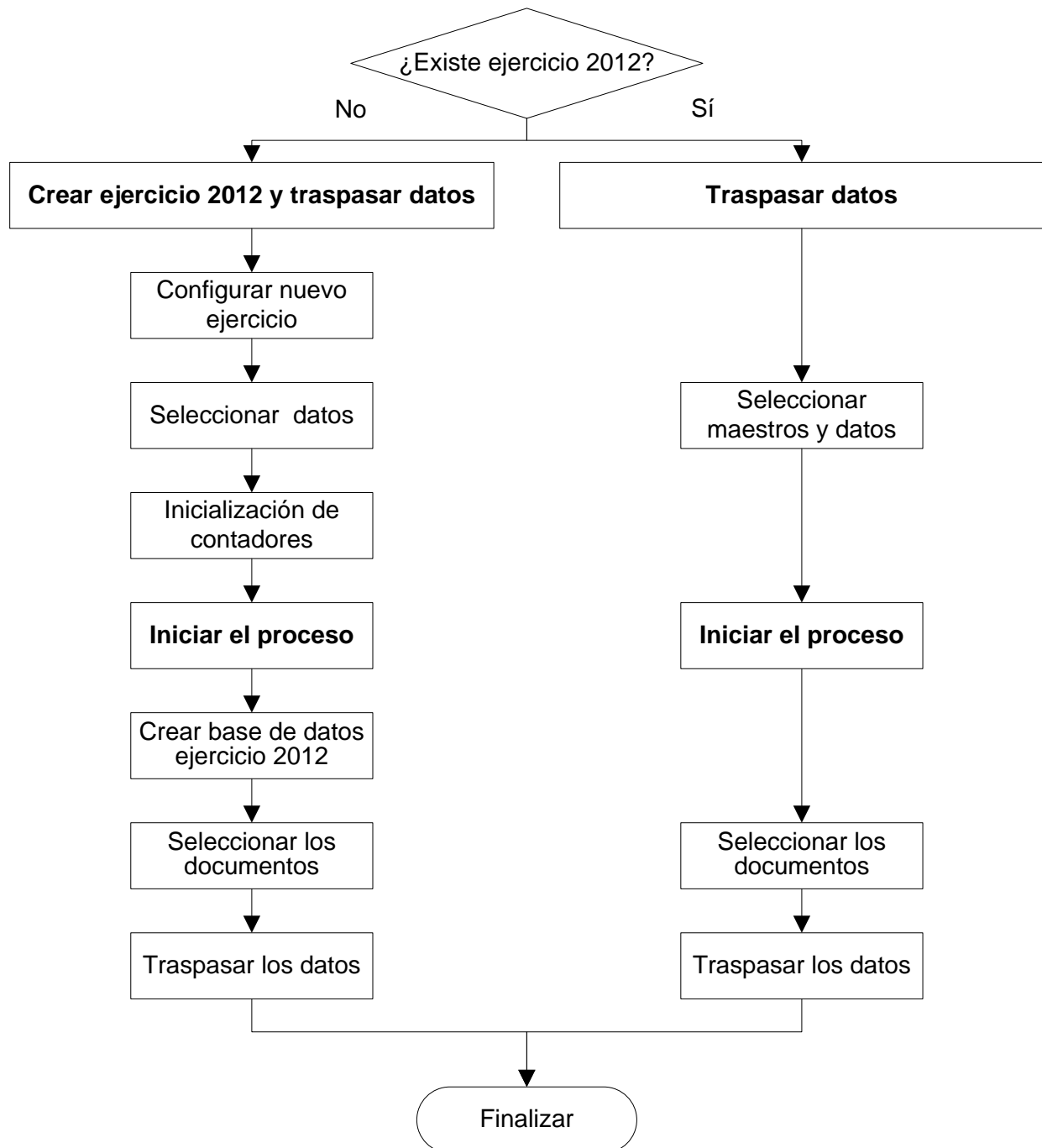
Figura 4. Esquema de la aplicación de apertura
